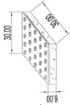
ТИП "А" - плоча упозорења
