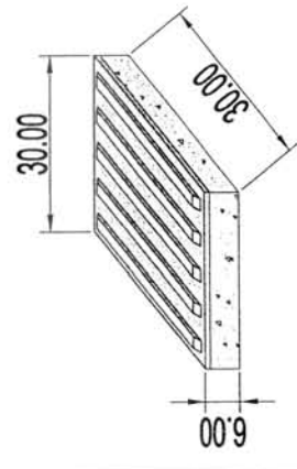
ТИП "Б" - плоча водилца за слепа и слабовиде
